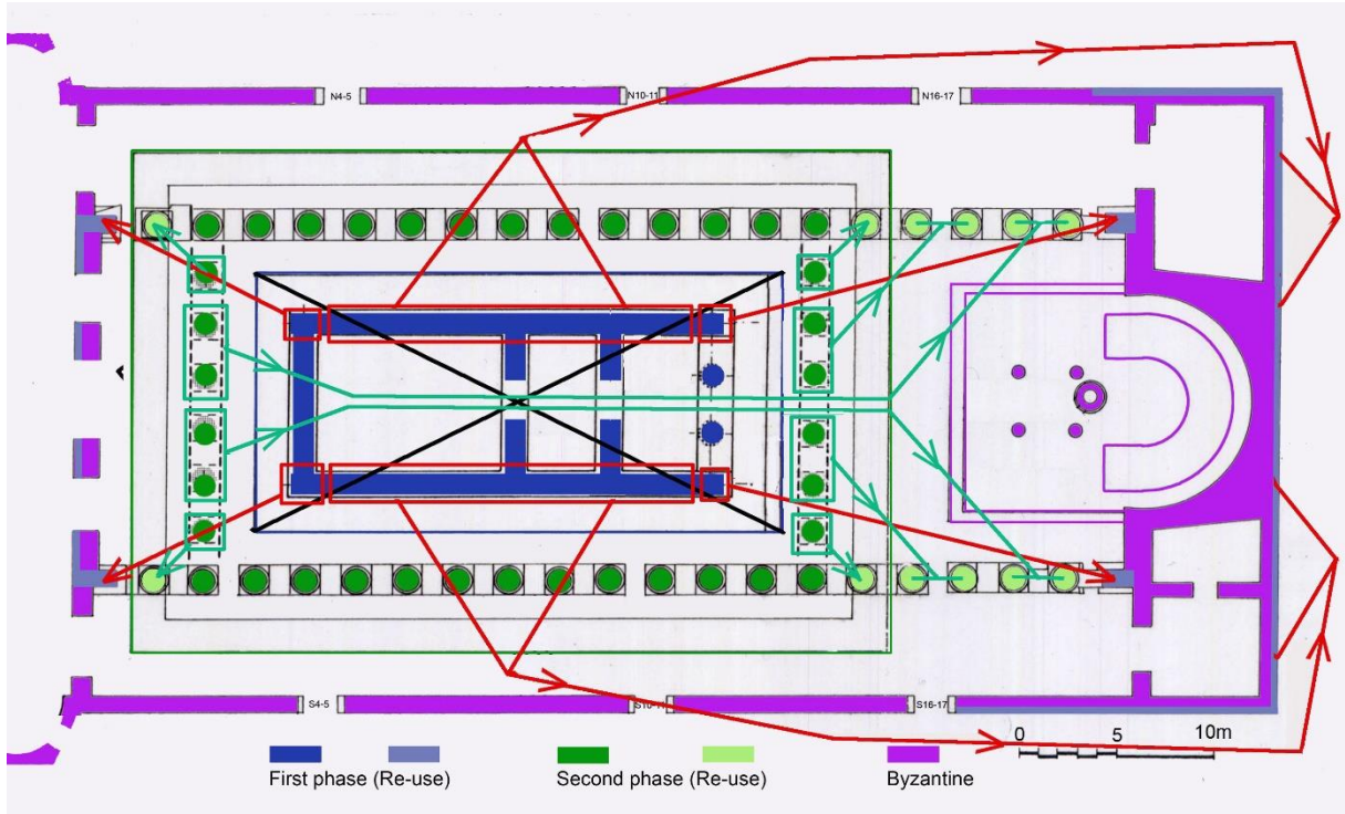
Res. 26: Tapınağın kiliseye dönüştürülmesi: Erken imparatorluk döneminde Aphrodite Tapınağı'ndaki blokların beşinci yüzyıl Hıristiyan katedralindeki mevcut konumlara hareketlerini gösteren Jim Coulton tarafından hazırlanan diyagram (2015).
